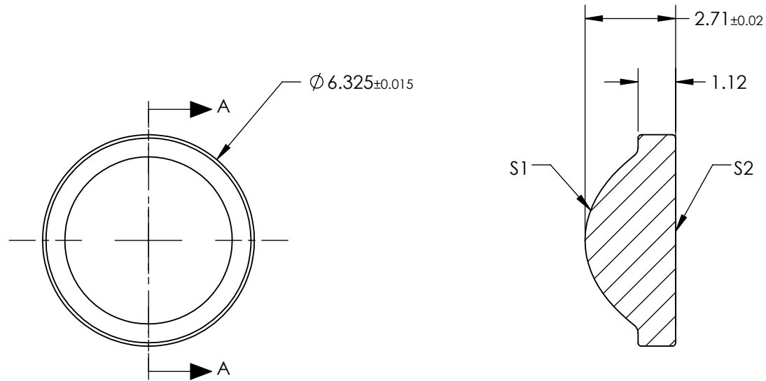
SECTION A-A
