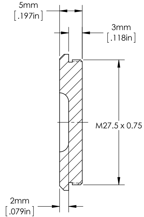
SECTION A-A
